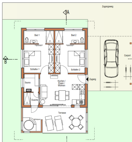
Grundriss, Quelle: Architekturbüro Kaiser
