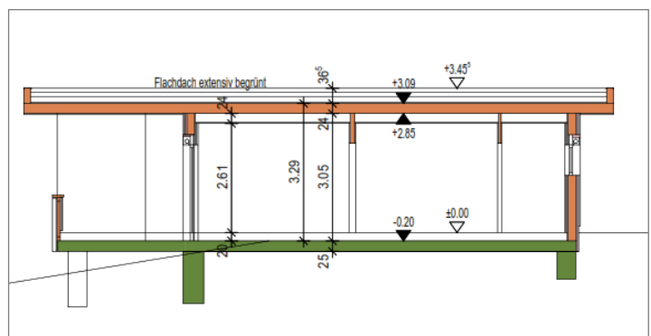
Schnitt A-A, Quelle: Architekturbüro Kaiser
